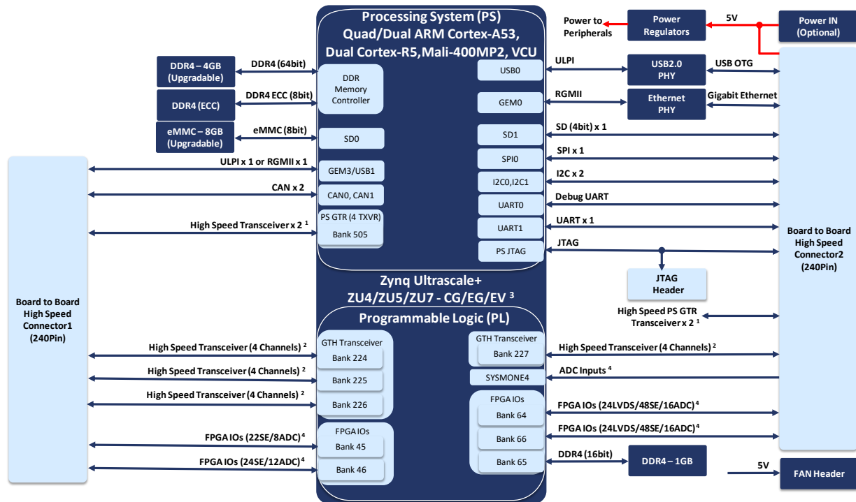
iW-RainboW-G30M – Zynq Ultrascale+ MPSoC SOM Block Diagram
