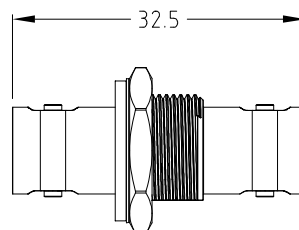
BNC INSERT
