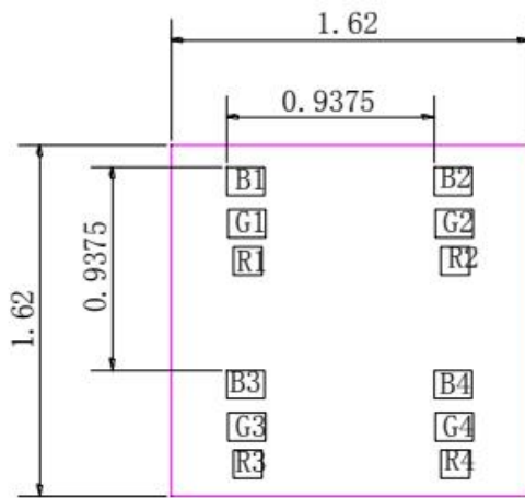
灯面正视图
