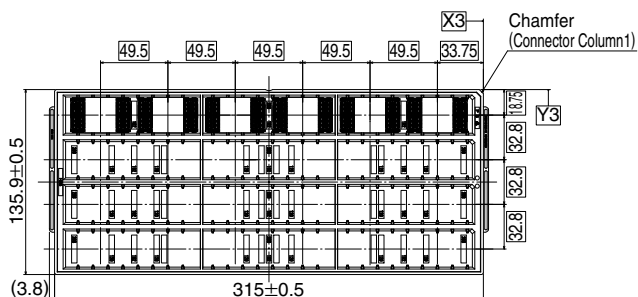
IT8MB-192S-BGA-***H
