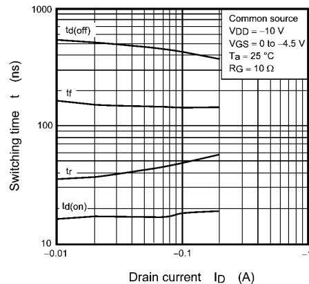
Fig. 7.10 t - I_D
