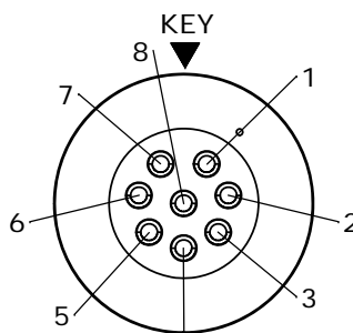
WIRING END W7282-8PG-P-300
