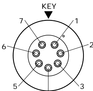
WIRING END W7282-7PG-P-300
