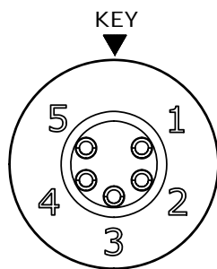
WIRING END W7282-5PG-P-300
