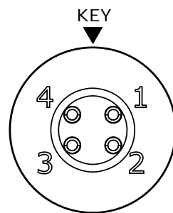
WIRING END W7282-4PG-P-300
