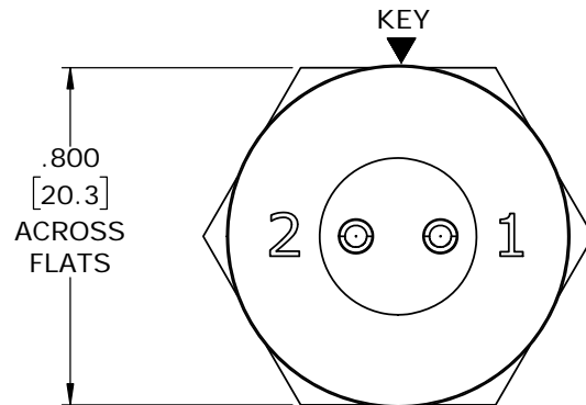
WIRING END W7282-2PG-P-300 SHOWN
