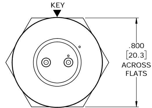
WIRING END W7281-2SG-P-3ES SHOWN
