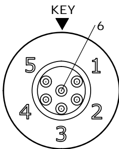
WIRING END W7281-6SG-P-3ES
