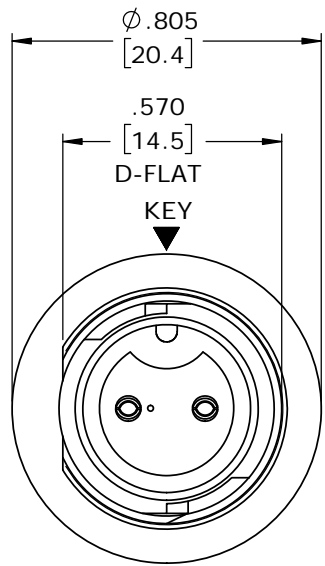
MATING FACE W7281-2SG-P-3ES SHOWN
