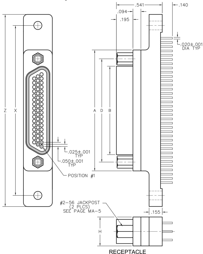
RECEPTACLE
