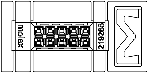
10 CKT
