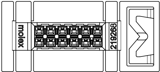
12 CKT
