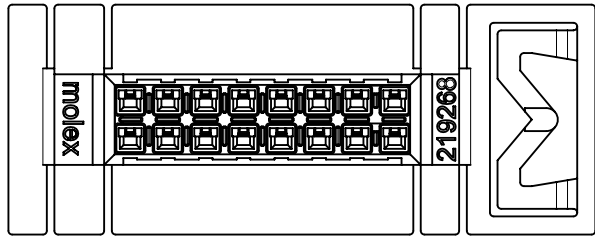
16 CKT
