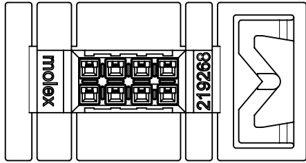
8 CKT
