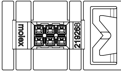
6 CKT
