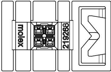
4 CKT
