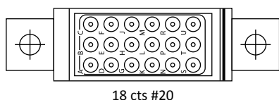
001758 202 02 A : 24,8 (.976) B : 22,5 (.885) Masse / Weight 28,0 g
