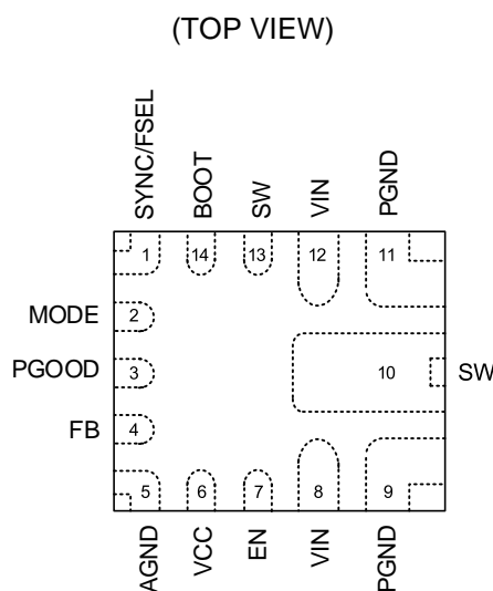
WQFN-14L 3x2.5 (FC)
