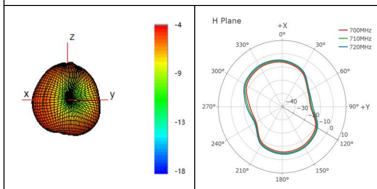
710 MHz
