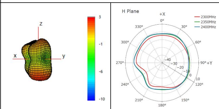
2350 MHz
