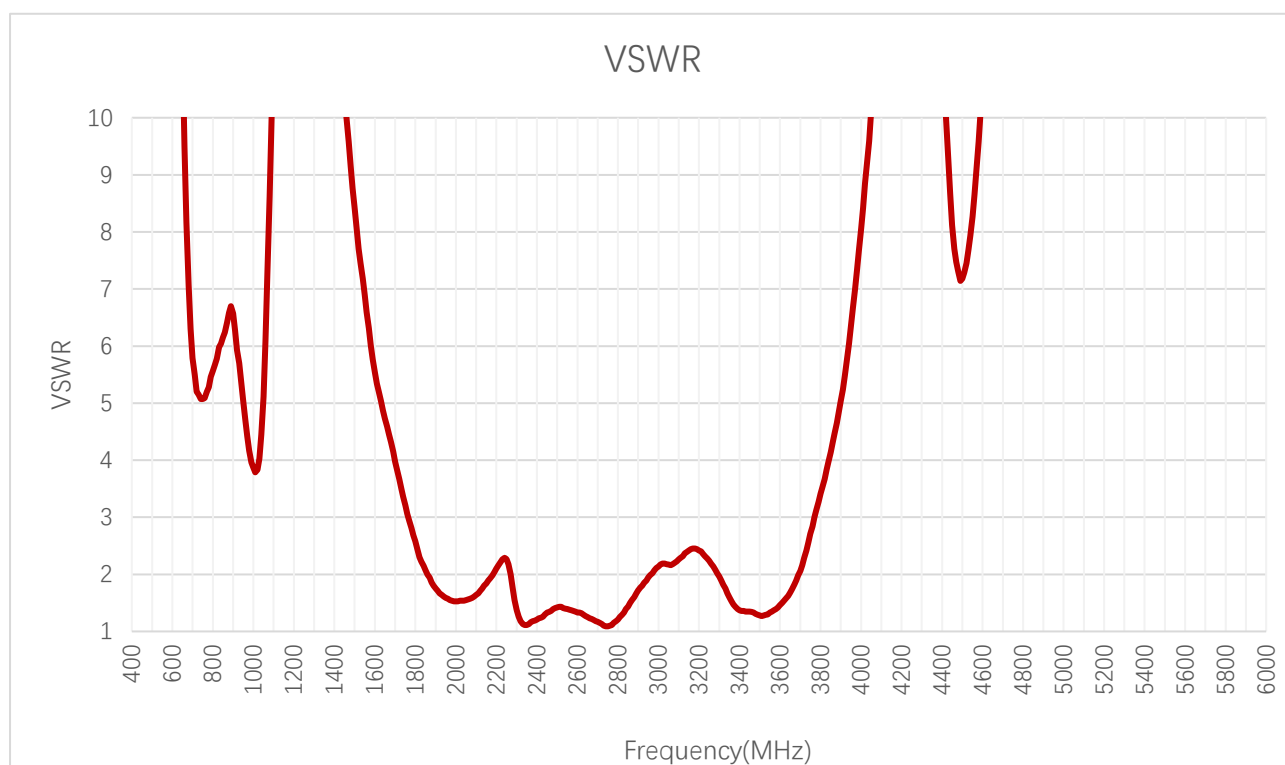
VSWR
