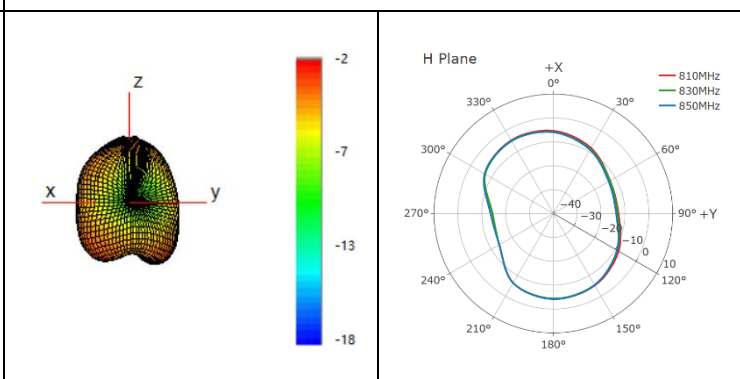
830 MHz
