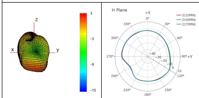
2140 MHz
