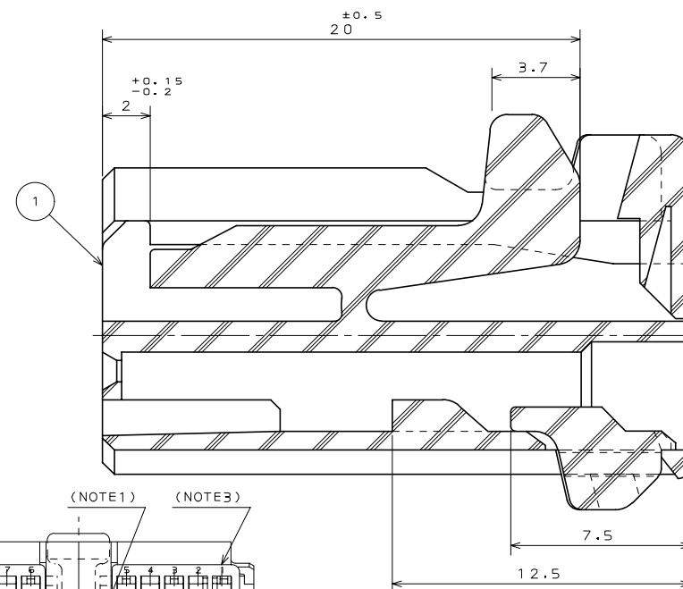
S E C T . A - A ( S C A L E 5 : 1 )
