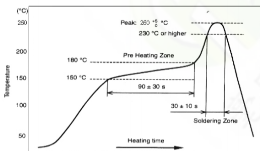
回流焊曲线图
