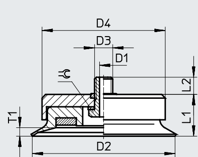
ESS-80/100-E
