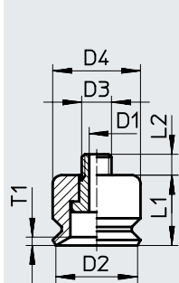
ESS-15-E
