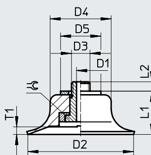
ESS-40/50/60-E
