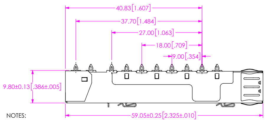
FIG 1 QSFP-C-1-1-S-F SHOWN
