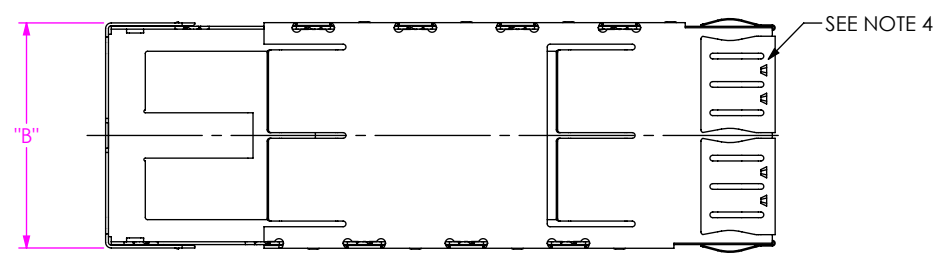
FIG 1 QSFP-C-1-1-S-F SHOWN
