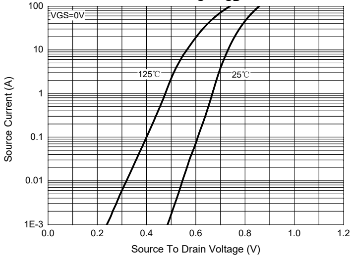
Fig.9 - I_S - V_{SD}
