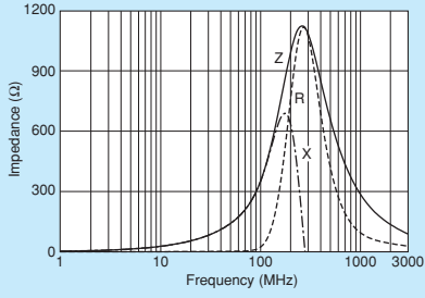
BLM21BB331SZ1/BLM21BB331SH1
