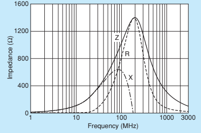
BLM15BX102SZ1
