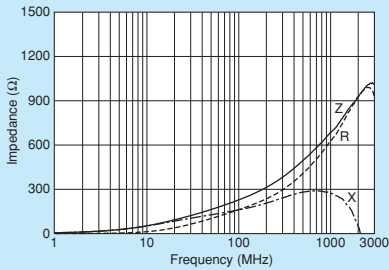
BLM15GG221SZ1
