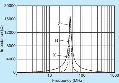
NFZ32BW650HZ11
