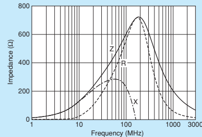
BLM15PX601SZ1
