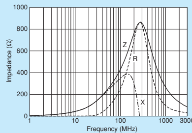
BLM18BD421SZ1/BLM18BD421SH1
