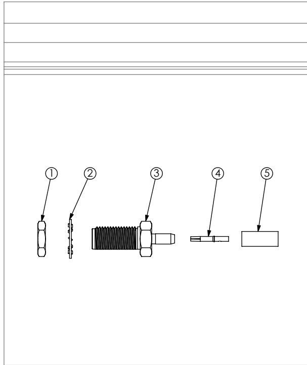
FIG 2 SMA-J-C-X-ST-BH1 SHOWN
