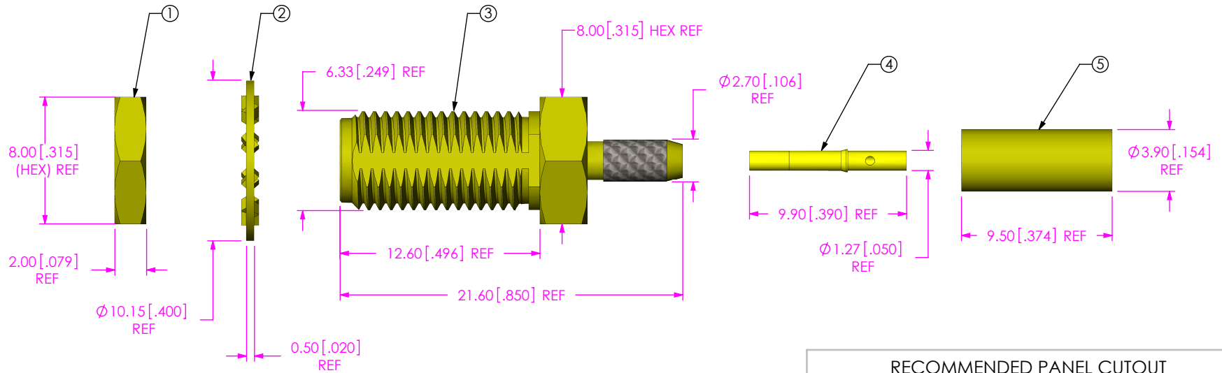
FIG1 SMA-J-C-X-ST-BH1 SHOWN
