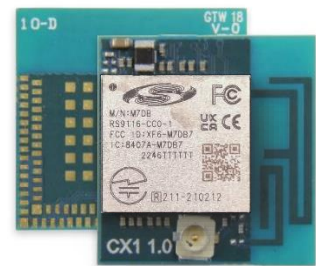
LGA Module (15 x 15.7 x 2.3) mm
