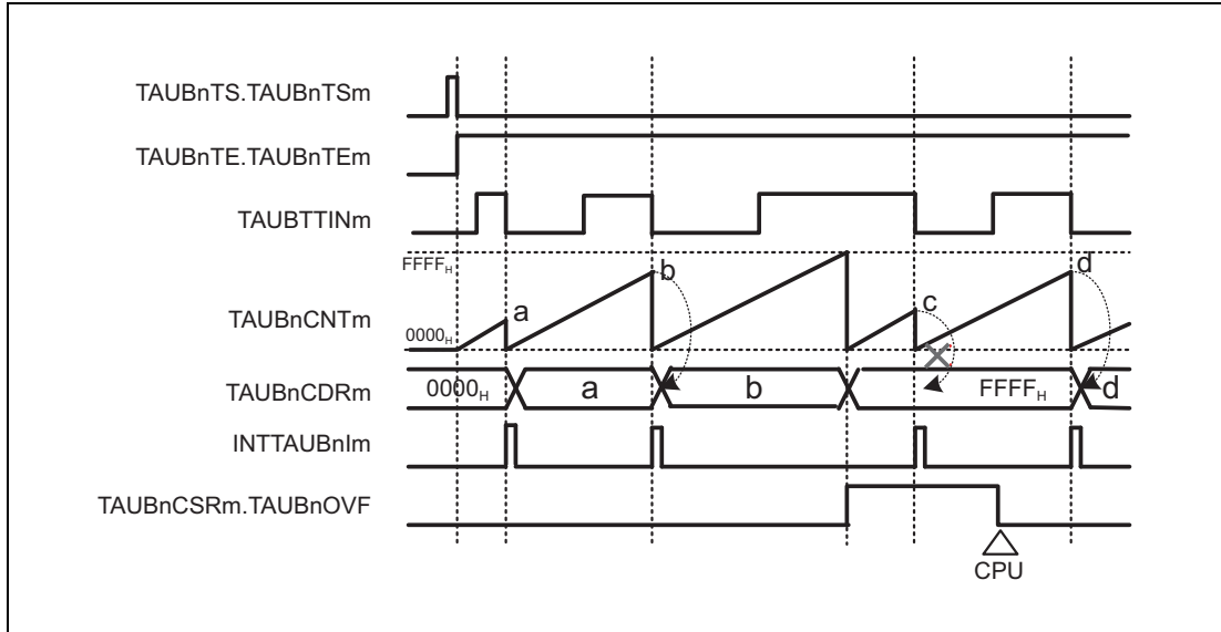
Figure 29.52 TAUBnCMORm.TAUBnCOS[1:0] = 11 B , TAUBnCMORm.TAUBnMD0 = 0, TAUBnCMURm.TAUBnTIS[1:0] = 00 B
