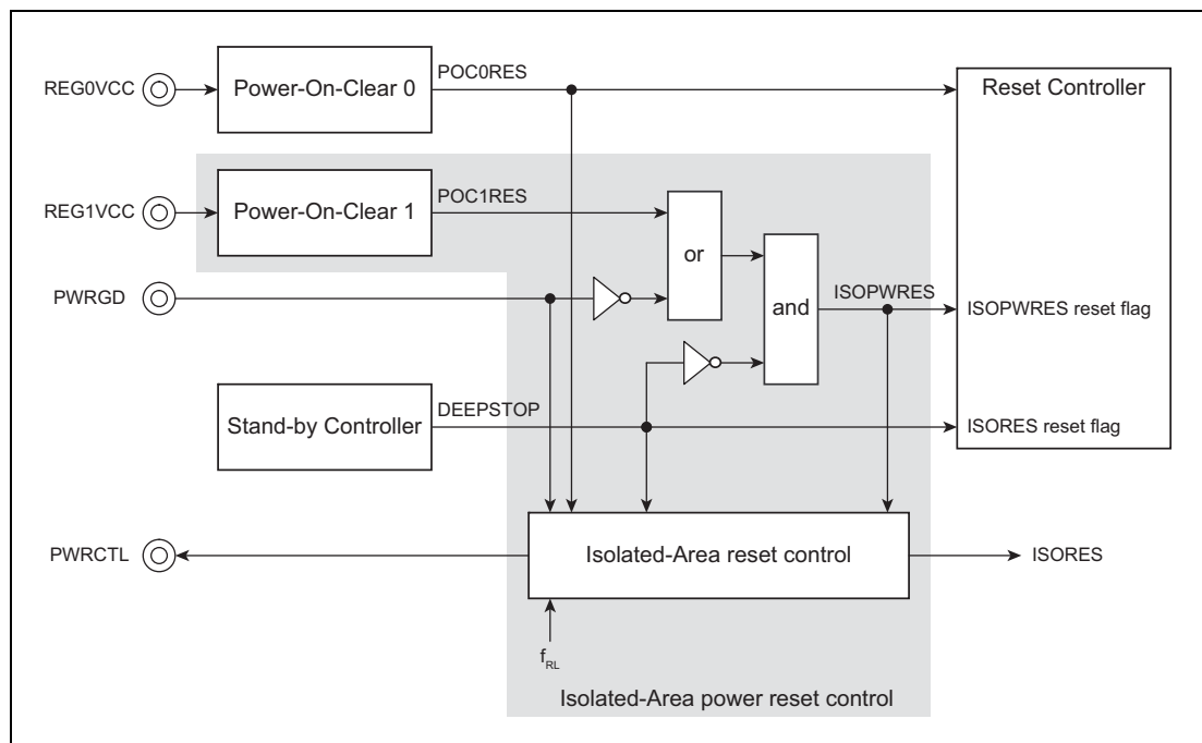
Figure 9.2 D1Lx, D1M1(H), D1M1-V2 and D1M1A Isolated-Area power reset
