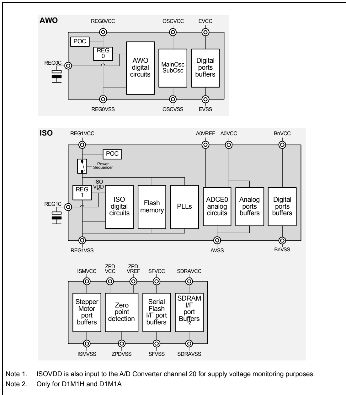
Figure 10.2 D1M1(H), D1M1-V2 and D1M1A power supply overview
