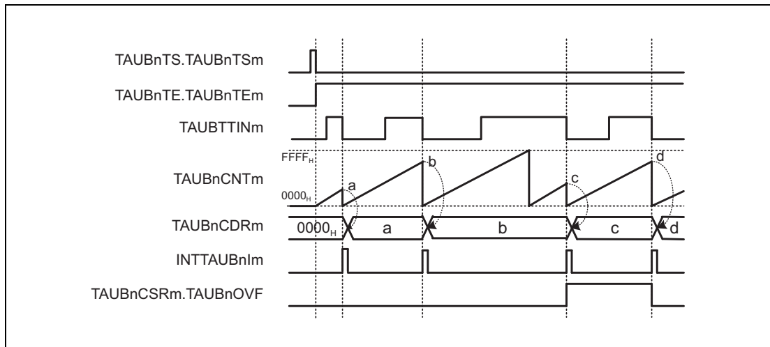
Figure 29.49 TAUBnCMORm.TAUBnCOS[1:0] = 00 B , TAUBnCMORm.TAUBnMD0 = 0, TAUBnCMURm.TAUBnTIS[1:0] = 00 B
