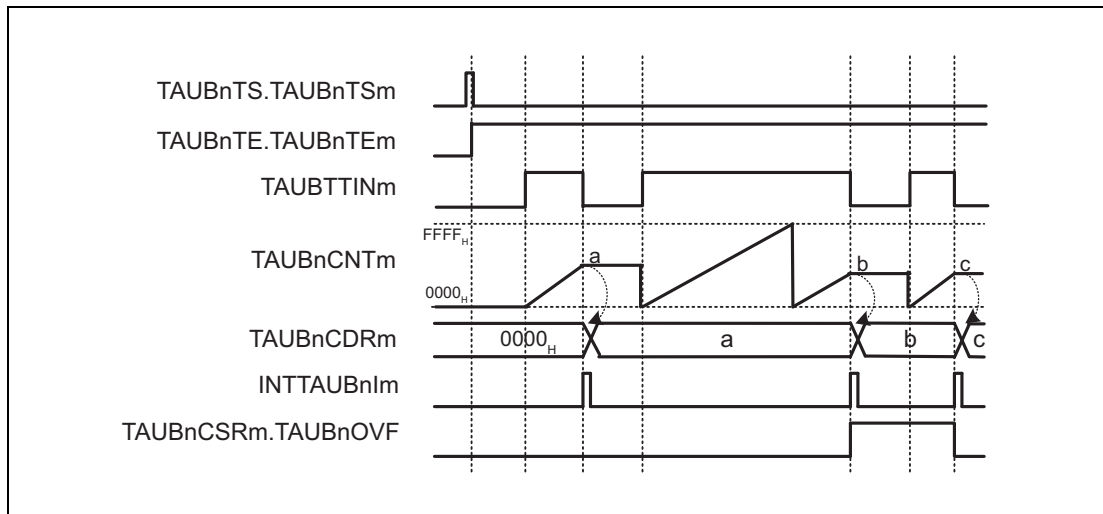
Figure 29.57 TAUBnCMORm.TAUBnCOS[1:0] = 00 B , TAUBnCMORm.TAUBnMD0 = 0, TAUBnCMURm.TAUBnTIS[1:0] = 11 B
