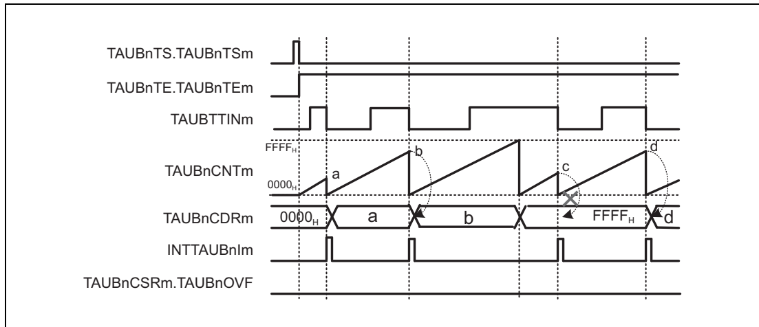
Figure 29.51 \text{TAUBnCMORm.TAUBnCOS}[1:0] = 10_{\text{B}} , \text{TAUBnCMORm.TAUBnMD0} = 0 , \text{TAUBnCMURm.TAUBnTIS}[1:0] = 00_{\text{B}}
