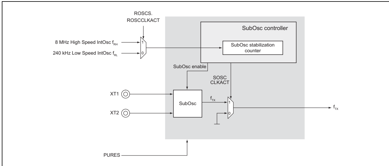
Figure 12.12 Sub Oscillator (SubOsc)
