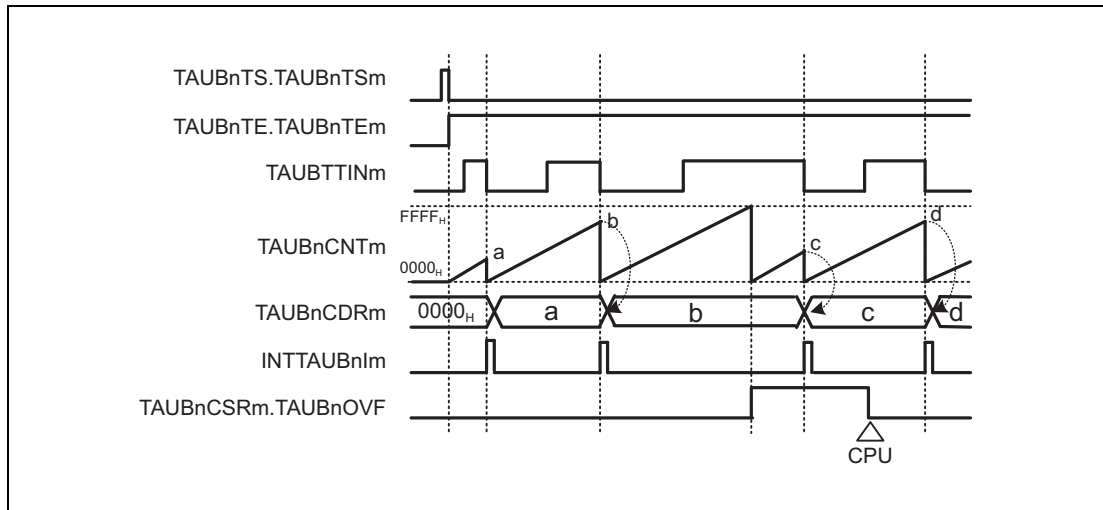
Figure 29.50 TAUBnCMORm.TAUBnCOS[1:0] = 01 B , TAUBnCMORm.TAUBnMD0 = 0, TAUBnCMURm.TAUBnTIS[1:0] = 00 B
