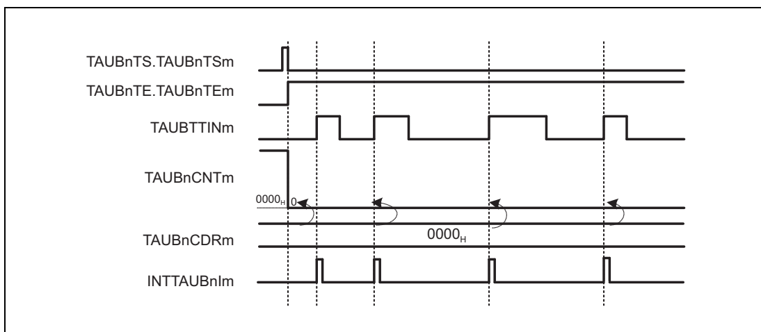
Figure 29.42 TAUBnCDRm = 0000 H , TAUBnCMURm.TAUBnTIS[1:0] = 01 B
