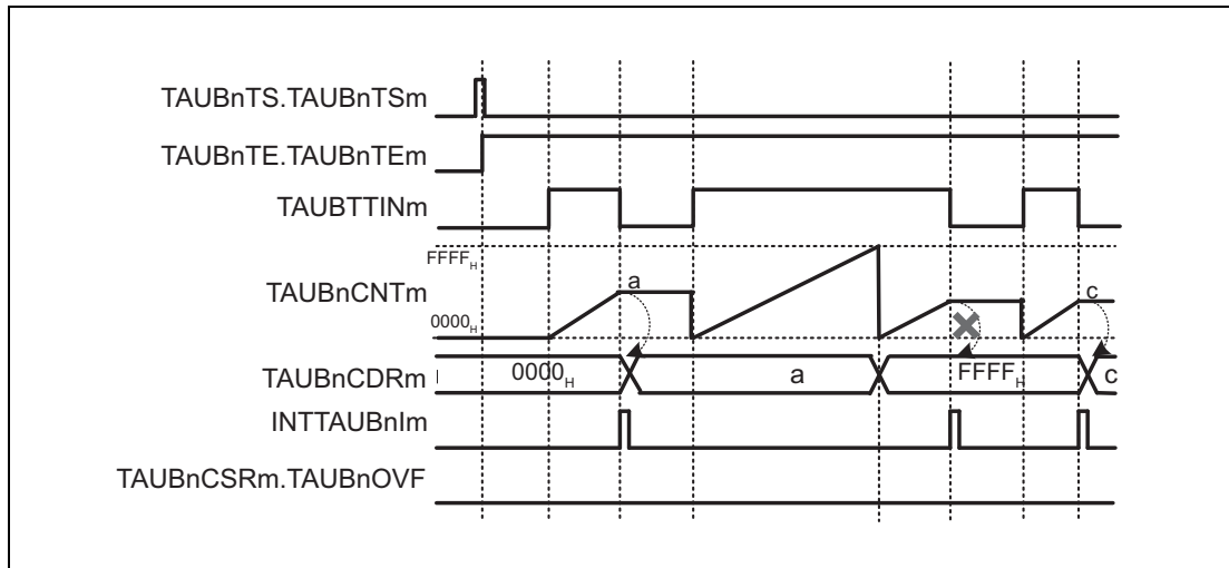
Figure 29.59 TAUBnCMORm.TAUBnCOS[1:0] = 10 B , TAUBnCMORm.TAUBnMD0 = 0, TAUBnCMURm.TAUBnTIS[1:0] = 11 B
