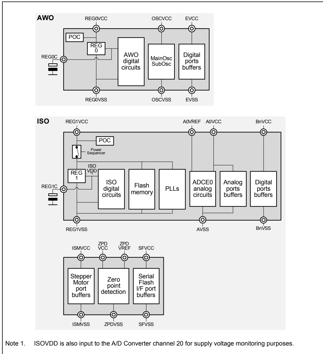
Figure 10.1 D1L1, D1L2(H) power supply overview
