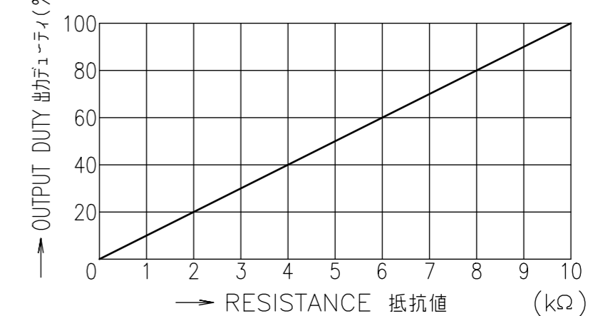
RESISTANCE - OUTPUT DUTY CHARACTERISTIC 抵抗値 - 出力デューティ特性例
