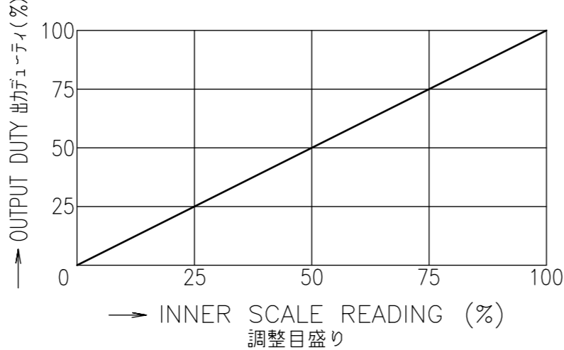
INNER SCALE READING - OUTPUT DUTY CHARACTERISTIC 調整目盛り - 出力デューティ特性例
