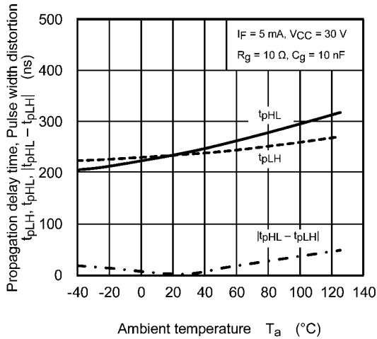
Fig. 12.2.13 t_{pHL} , t_{pLH} , |t_{pHL}-t_{pLH}| - T_a
