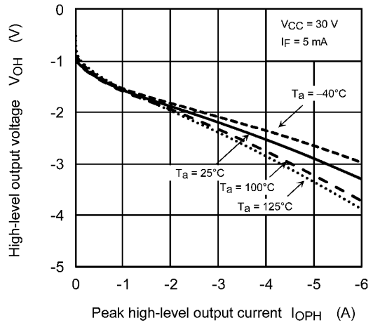
Fig. 12.2.10 VOH - IOPH
